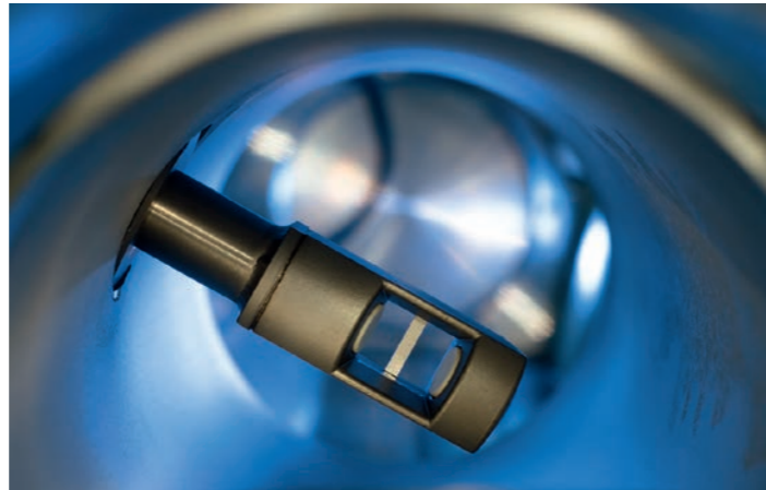
Sensorik für die Tabakgeschwindigkeit in der Zigarettenproduktionslinie PROTOS-M5
